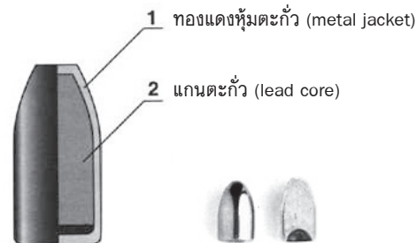
ภาพที่ 1.6 แสดงโครงสร้างองค์ประกอบของลูกกระสุนปืนชนิดทองแดงหุ้มตะกั่ว ( http://www.world.guns.ru ,13 มีนาคม 2553)
