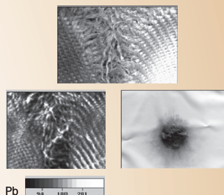
ภาพที่ 2.5 แสดงการเปรียบเทียบผลการวิเคราะห์หาธาตุตะกั่ว (Pb;Lead) บนเป่ายิงทดสอบในระยะยิงกดติดเป้า (Contact) ด้วยเทคนิค X-ray fluorescence Spectroscopy (XRF) และเทคนิค Sodium rhodizonate test
