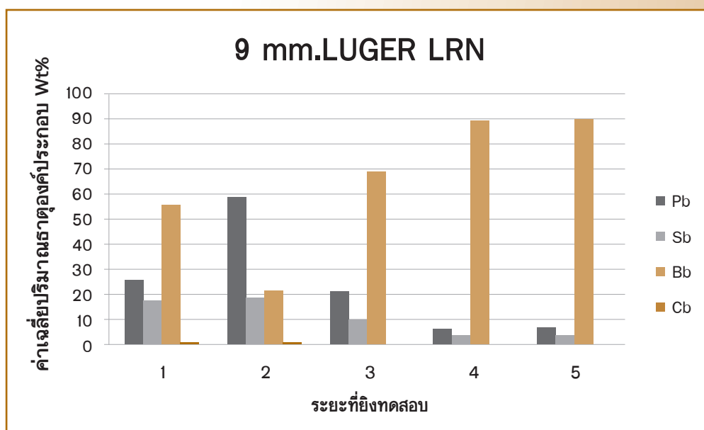
กราฟที่ 2.1 แสดงความสัมพันธ์ของธาตุองค์ประกอบสำคัญที่มาจากการยิงปืนต่อระยะในการยิงปืนกรณีปืนพกเซมิออโตเมติก ขนาด 9 มม. LUGER ด้วยลูกกระสุนปืนออโตเมติก ขนาด 9 มม. LUGER ชนิด LRN (Lead Round Nose)
