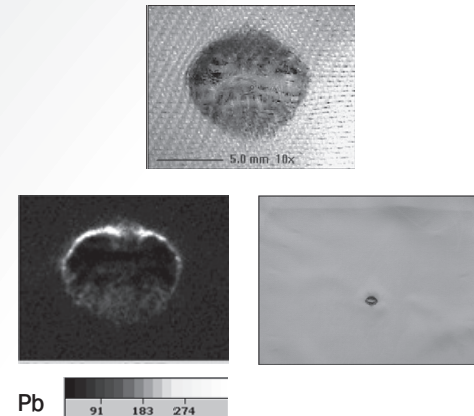
ภาพที่ 2.9 แสดงการเปรียบเทียบผลการวิเคราะห์หาธาตุตะกั่ว (Pb;Lead) บนเป้ายิงทดสอบ ในระยะ 3.5 ฟุต จากปลายลำกล้อง ด้วยเทคนิค X-ray fluorescence Spectroscopy (XRF) และเทคนิค Sodium rhodizonate test
