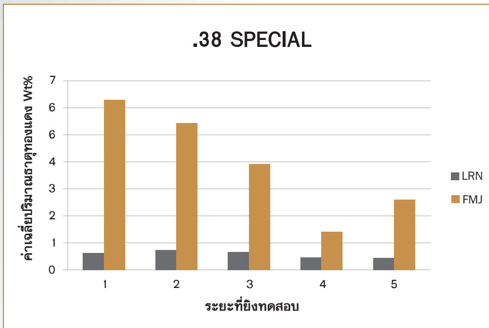
กราฟที่ 2.6 แสดงผลการเปรียบเทียบค่าเฉลี่ยปริมาณธาตุทองแดงที่ตรวจพบในแต่ละระยะยิงทดสอบปืนพกรีวอลเวอร์ ขนาด .38 SPECIAL ลูกกระสุนปืนชนิด LRN (Lead Round Nose) และ FMJ (Full Metal Jacket)
