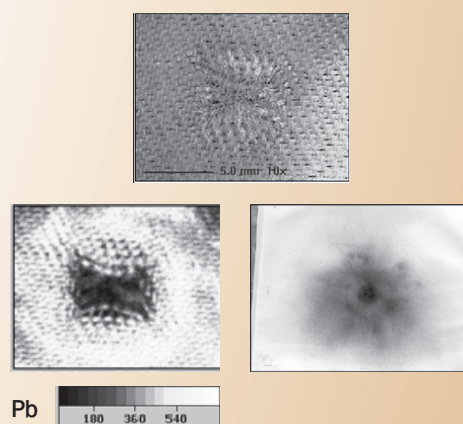
ภาพที่ 2.6 แสดงการเปรียบเทียบผลการวิเคราะห์หาธาตุตะกั่ว (Pb;Lead) บนเป่ายิงทดสอบในระยะประชิด (Near Contact) 1-4 นิ้วจากปลายลำกล้อง ด้วยเทคนิค X-ray fluorescence Spectroscopy (XRF) และเทคนิค Sodium rhodizonate test
