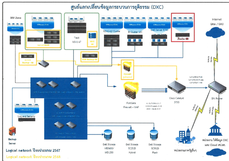
(ภาพแสดงแผนผังการติดตั้งระบบ Network และ VMware ปีงบประมาณ ๒๕๖๘)
